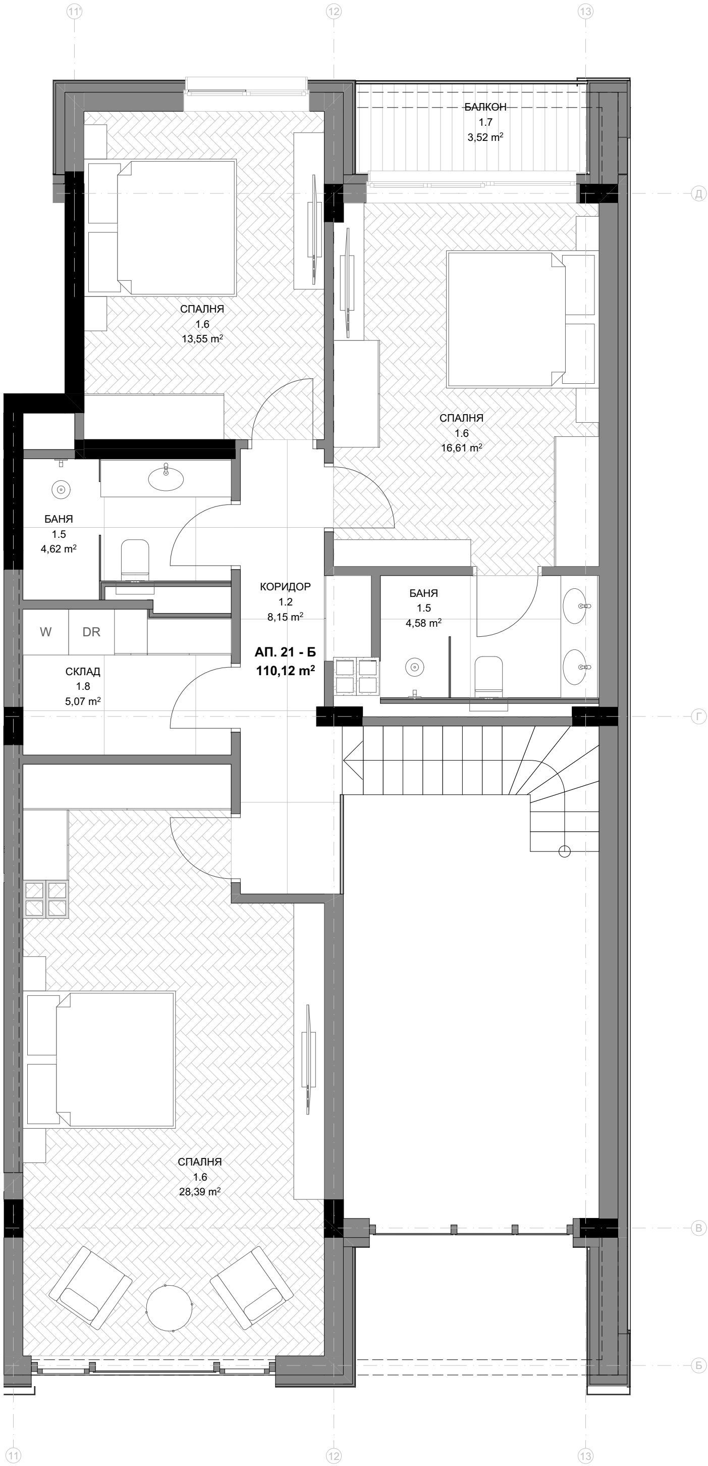
СЕКЦИЯ Б - НИВО 20,23 - АП. 21
